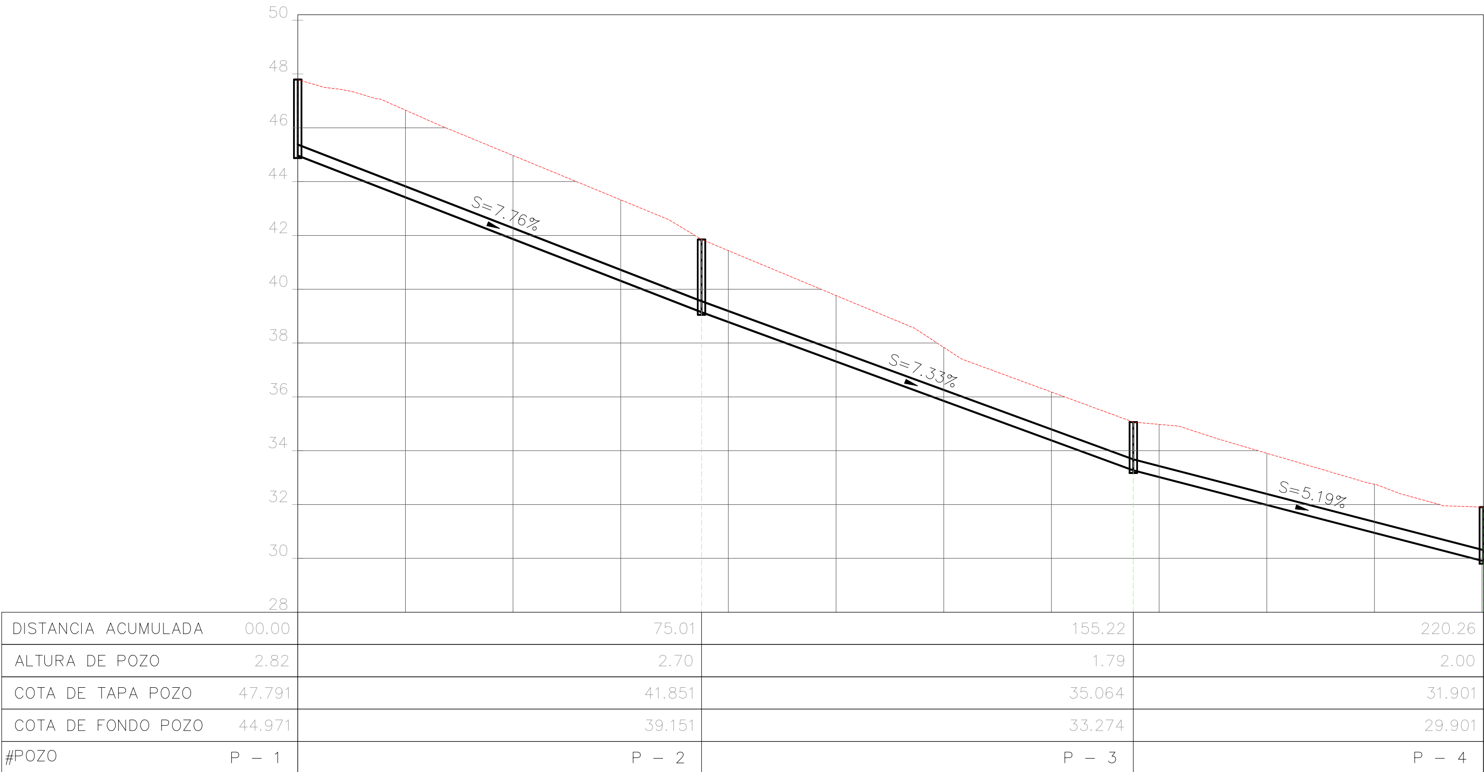
Perfil: 3er. Callejon 22 NO
