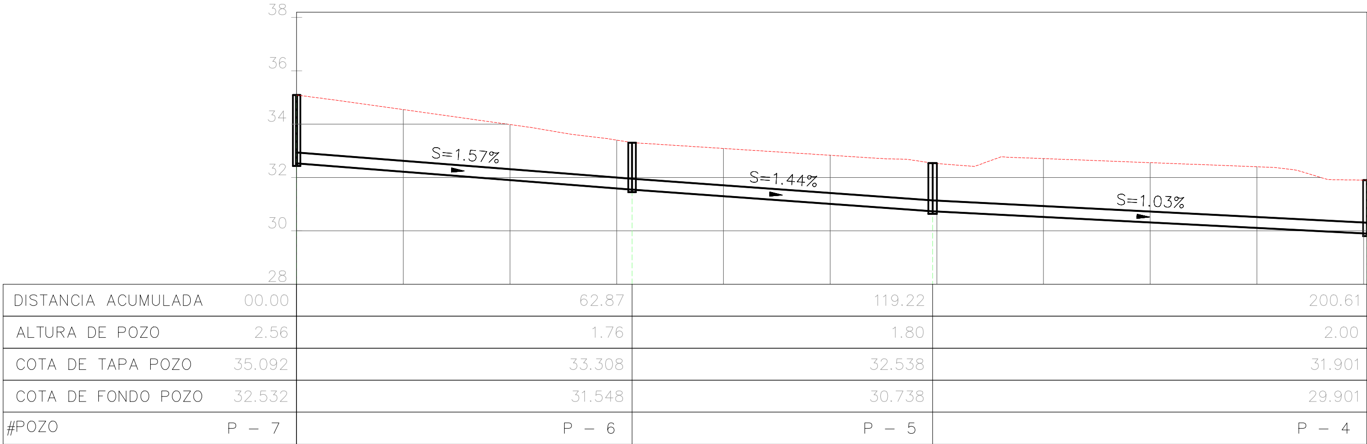
Perfil: Avenida 42A NO
