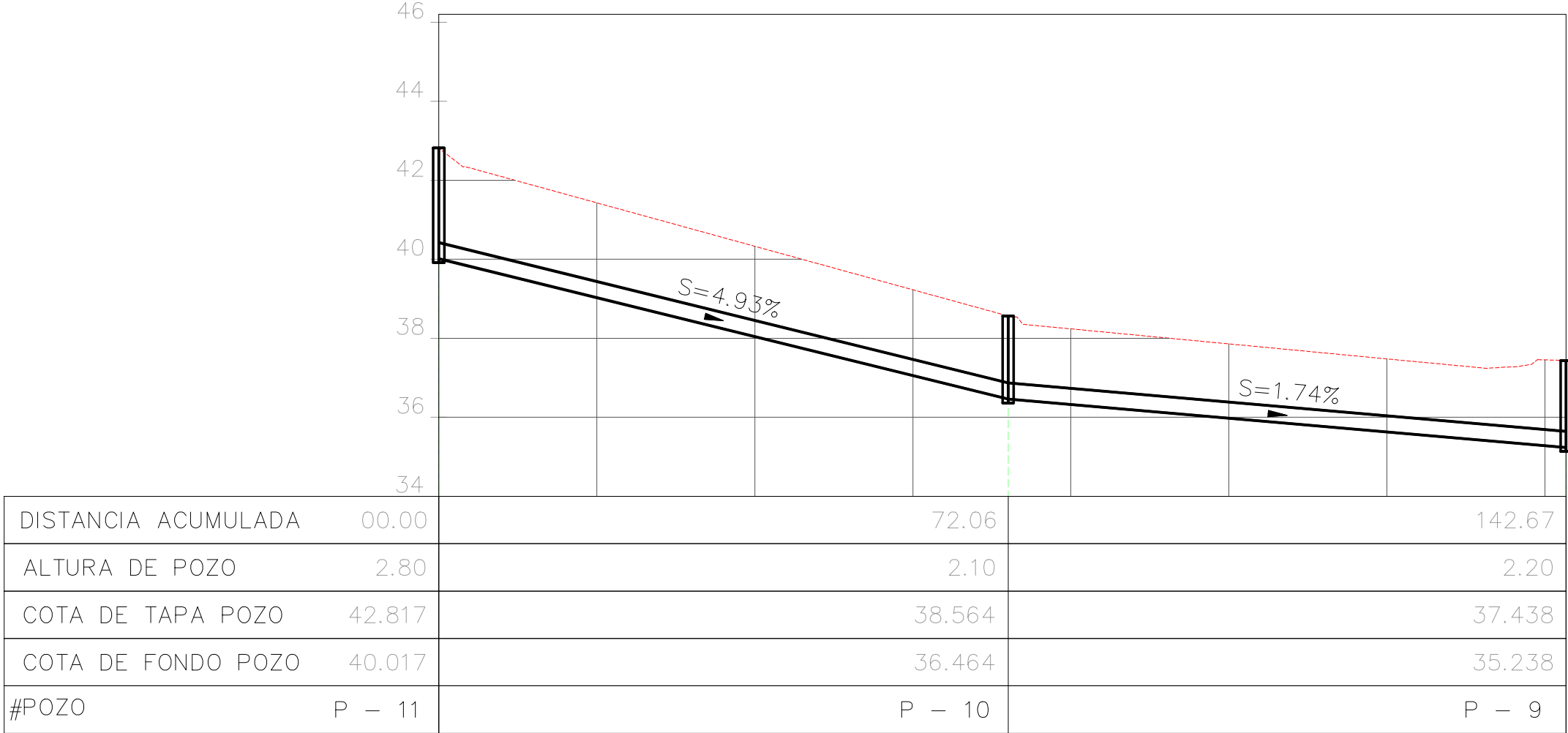
Perfil: 8° Pasaje 42A
