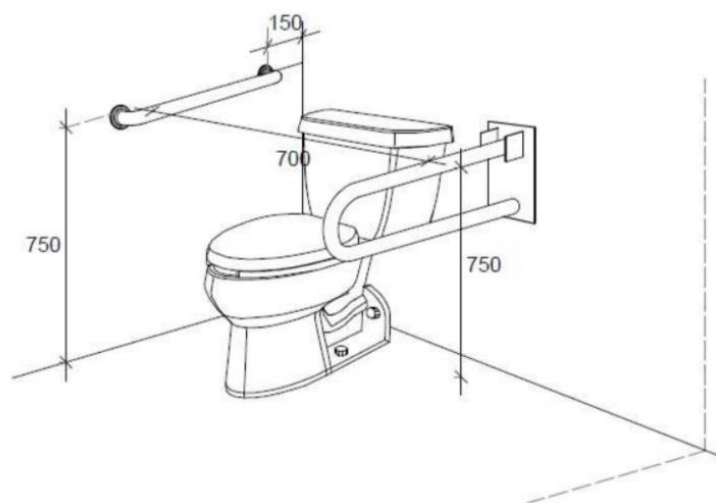
Isometría
