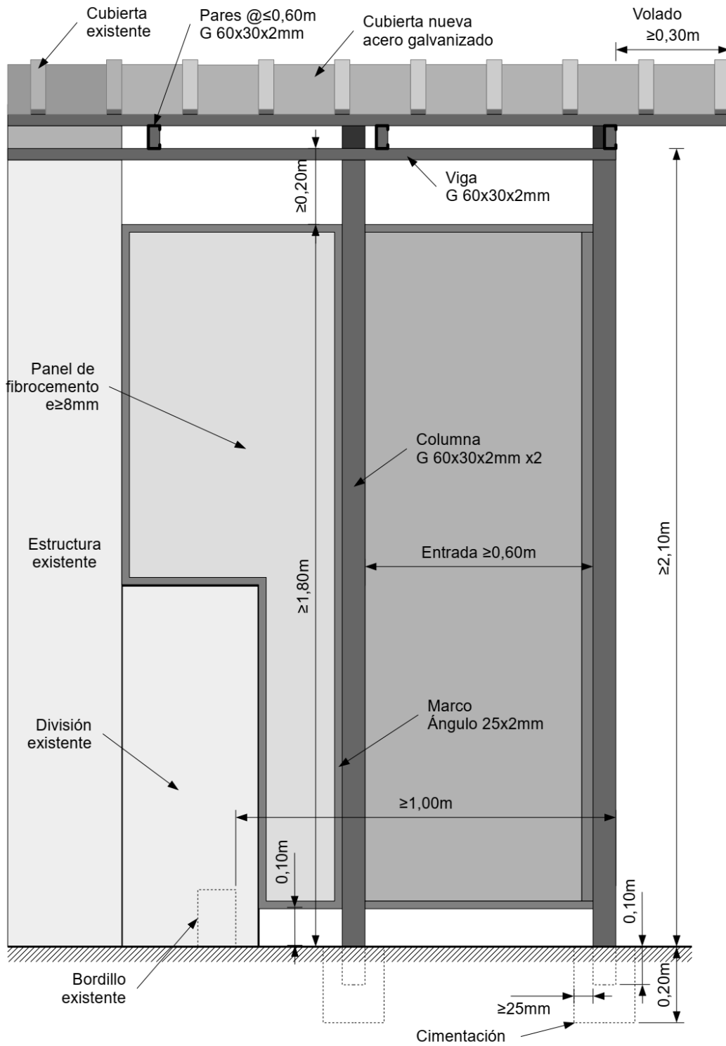
Vista lateral
